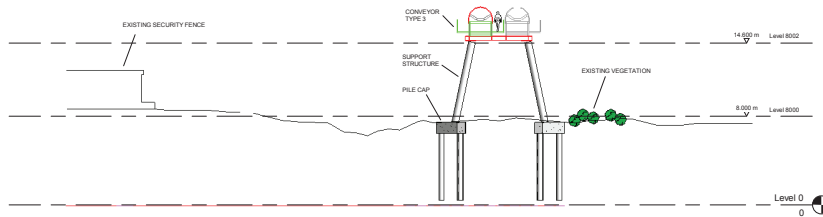
Section D-D 1:200
