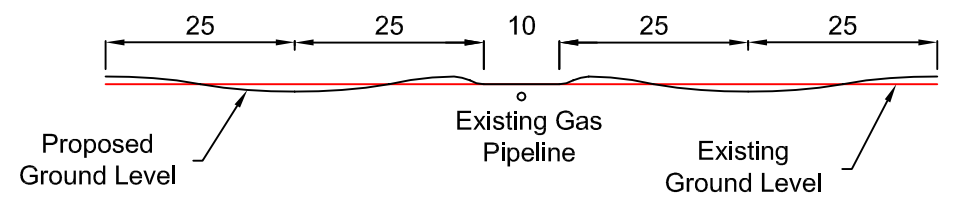
Section A - A Scale 1:1,000 @A3
