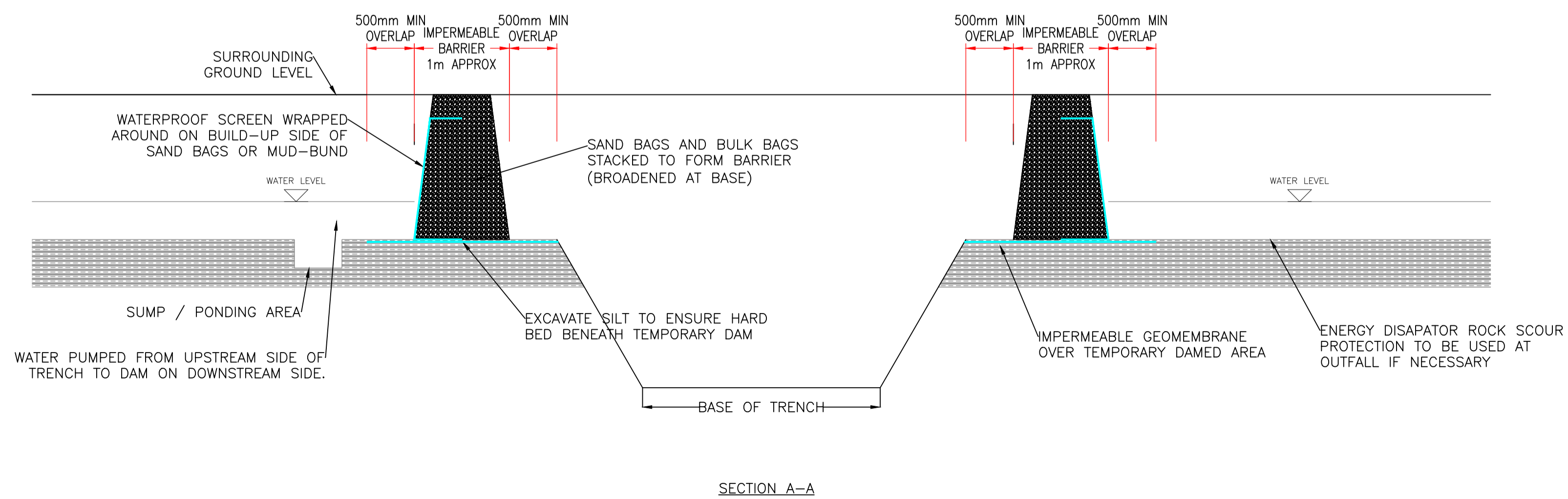
SECTION A-A
