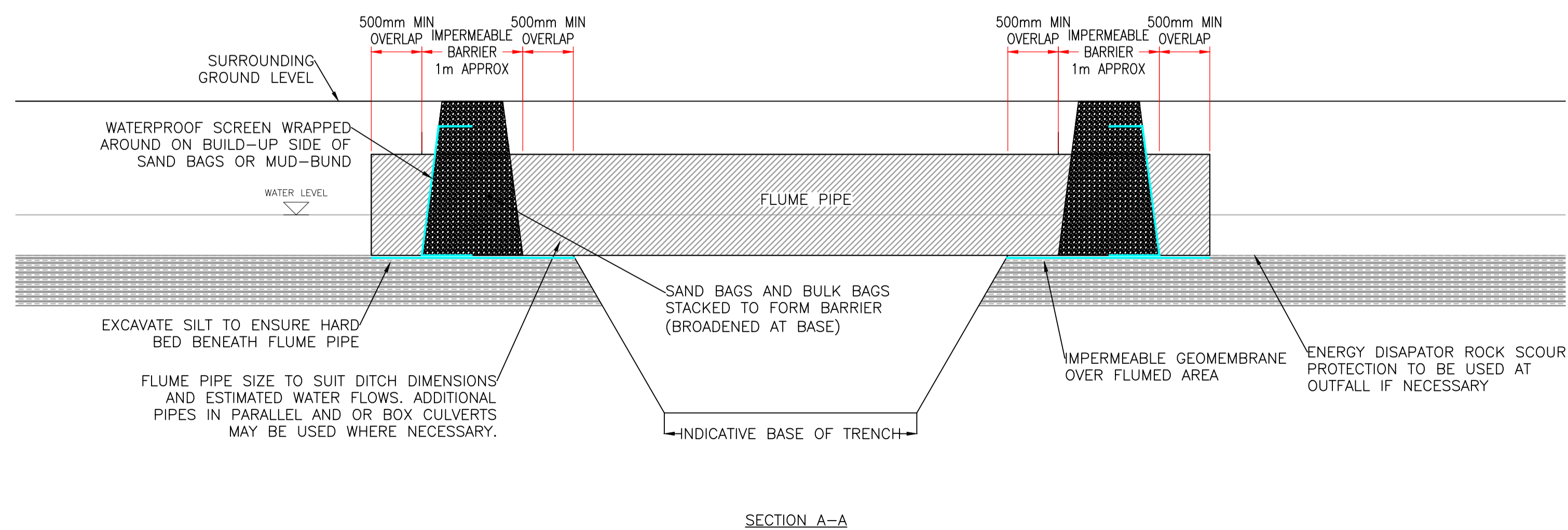
SECTION A-A
